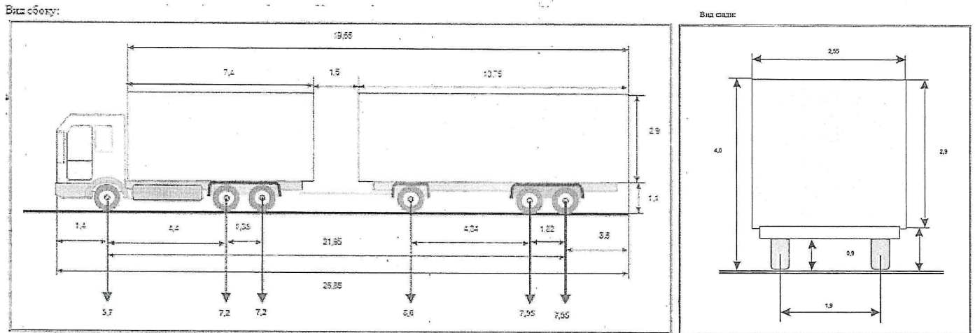
СХЕМА тяжеловесного и (или) крупногабаритного автопоезда
